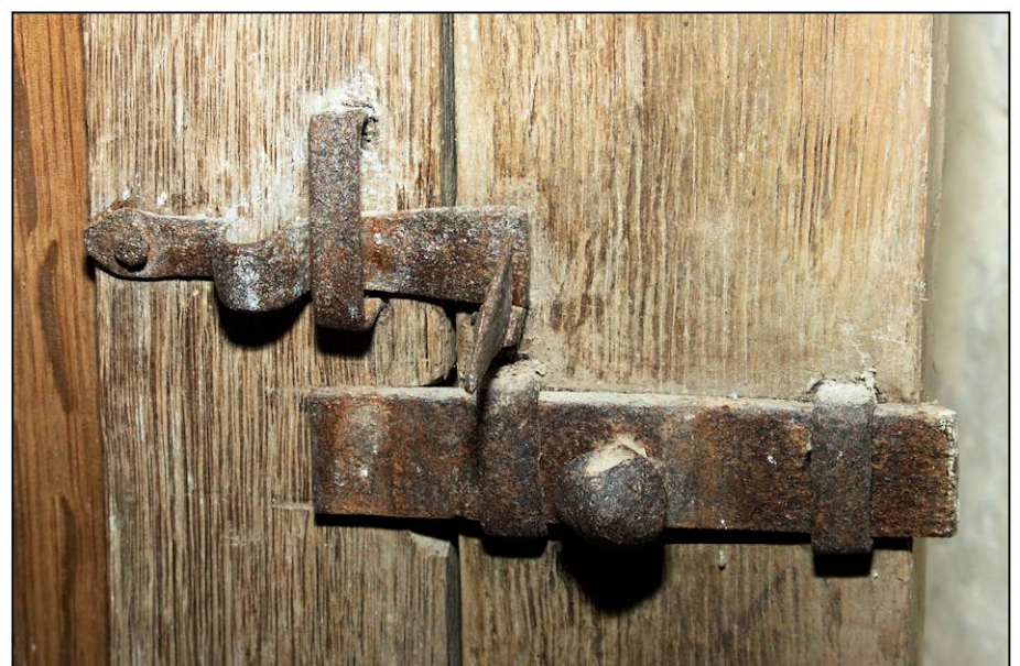
Fig. 2.6. Vantaill et volet supérieurs (loquet et targette)
