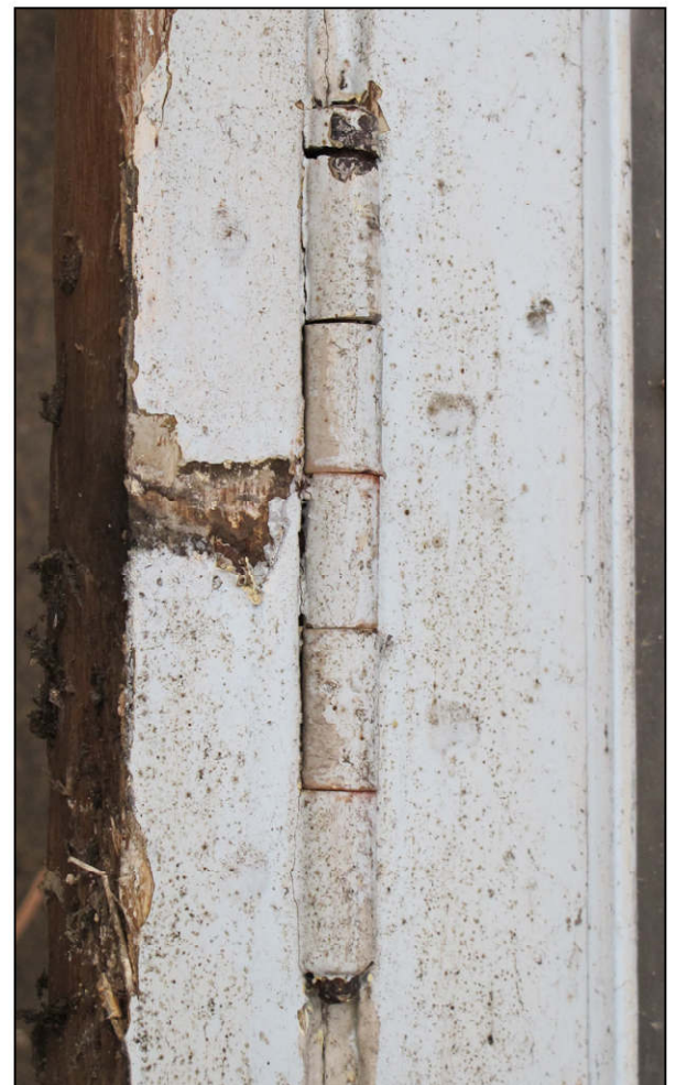
Fig. 6.6. Fiche à broche amovible (F)
