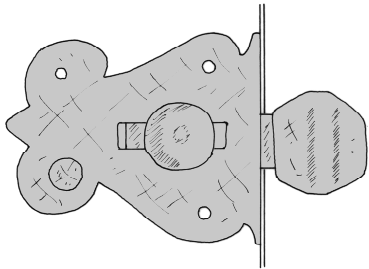
targette enclouonnée
