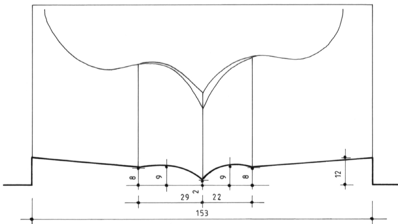
Fig. E.3 – Détail d'un panneau à plis de serviette (vantail de porte B).
