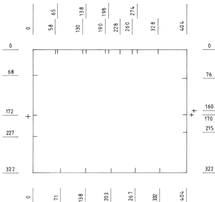
Fig. E.2 – Compartiment vitré du châssis de fenêtre (cotes en fond de feuillures) – emplacement des clous et de la vergette horizontale.
