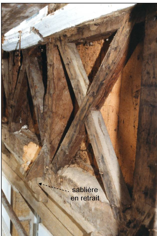
Fig. 1.4. Travées 2 et 3
