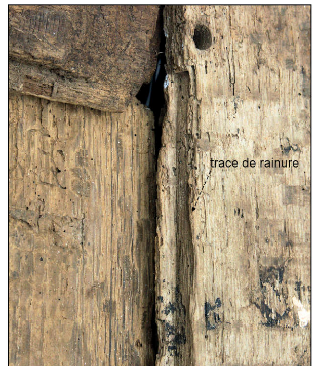
Fig. 3.5. Traverse haute / battant gauche (ext.)
