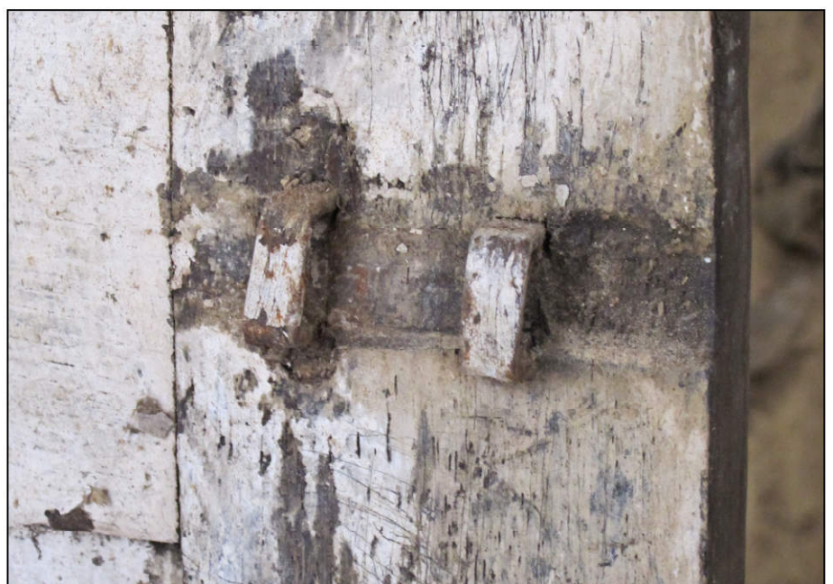
Fig. 2.6. Volet inférieur gauche / brides du pêne de la targette
