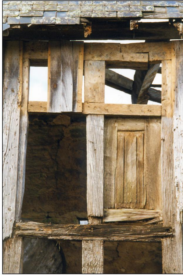
Fig. 2.2. Fenêtre / élévation extérieure
