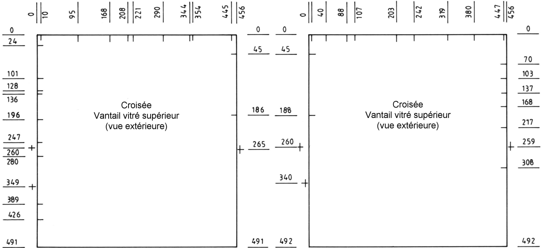
Emplacements des clous et des vergettes des vitreries
