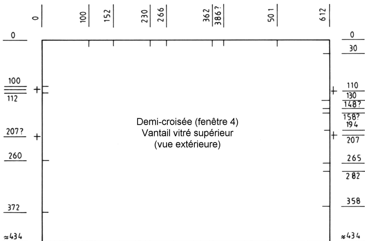
Emplacements des clous et des vergettes des vitreries
